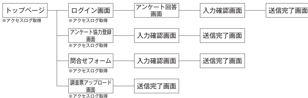
図表3 Webアンケートサイトの構成
